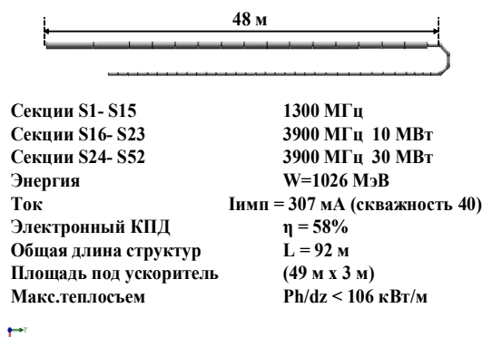
Рис.1. Компоновка двухчастотного (1300-3900 MHz) УЛОВ-1.0 ГэВ
